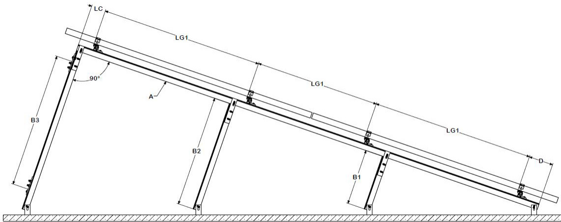
Figura 2: Dimensiones de ensamble para el sistema CrossRail Tilt-Up Multi-Row 1 Fila.
