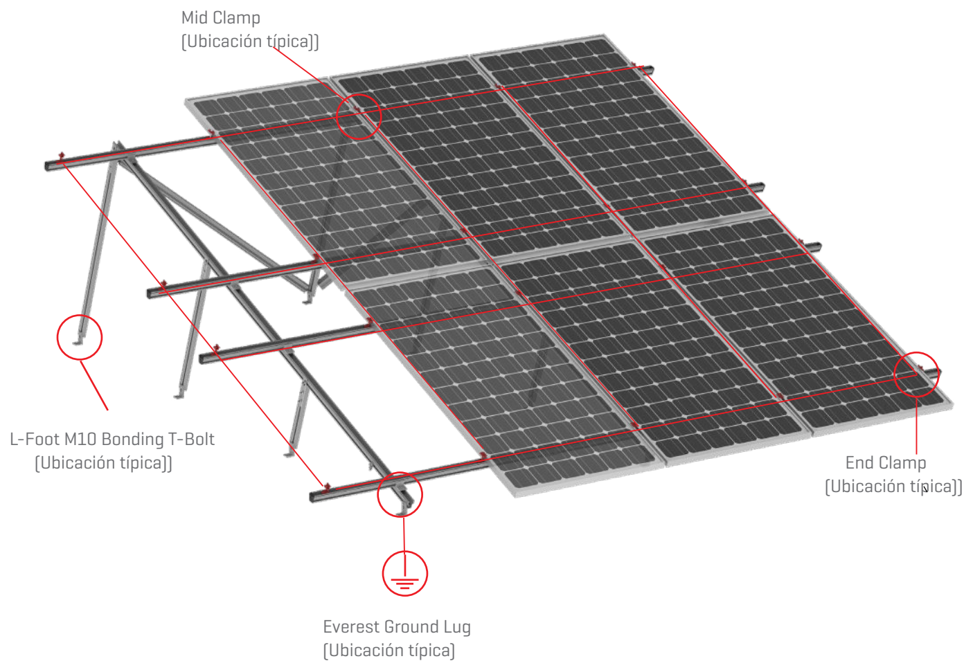
Figura 1: Conexión a tierra a través de Everest Ground Lug mostrado en rojo. Para ciertas regulaciones locales, las conexiones de enlace y conexión a tierra se identifican en ubicaciones típicas.
